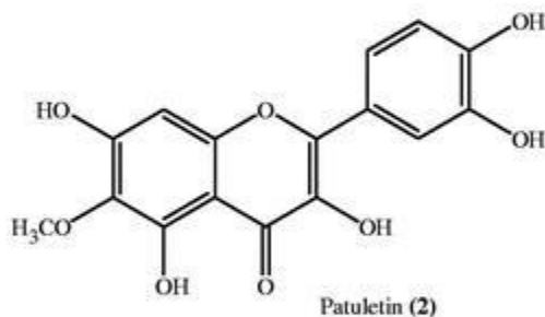
Patuletin (2)
