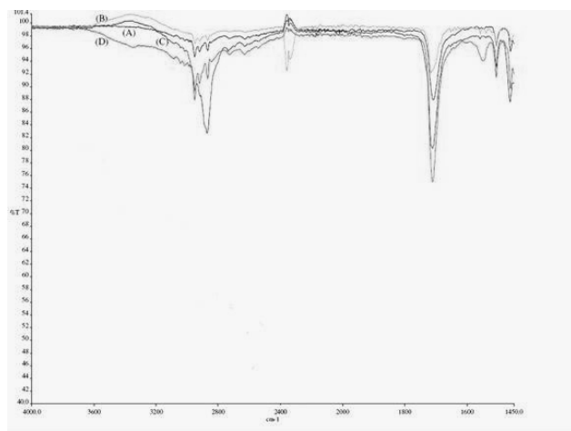
Fig. 3: FT-IR spectra of ibuprofen formulations: (A) pure ibuprofen (control), B) spray dried ibuprofen, (C) spray dried ibuprofen/Poloxamer 127 (1:1), (D) spray chilled ibuprofen.
